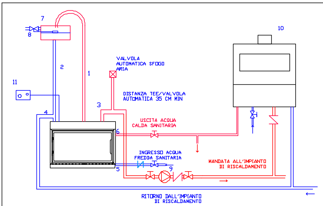
Figura 7 SCHEMA DI COLLEGAMENTO MERCURY 35 AD IMPIANTO TRADIZIONALE
