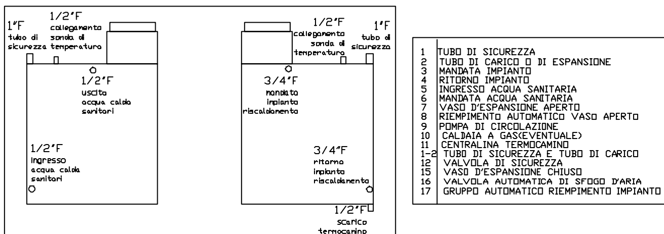
Figura 7 POSIZIONE E DIAMETRO DEI RACCORDI DI COLLEGAMENTO ALL'IMPIANTO
