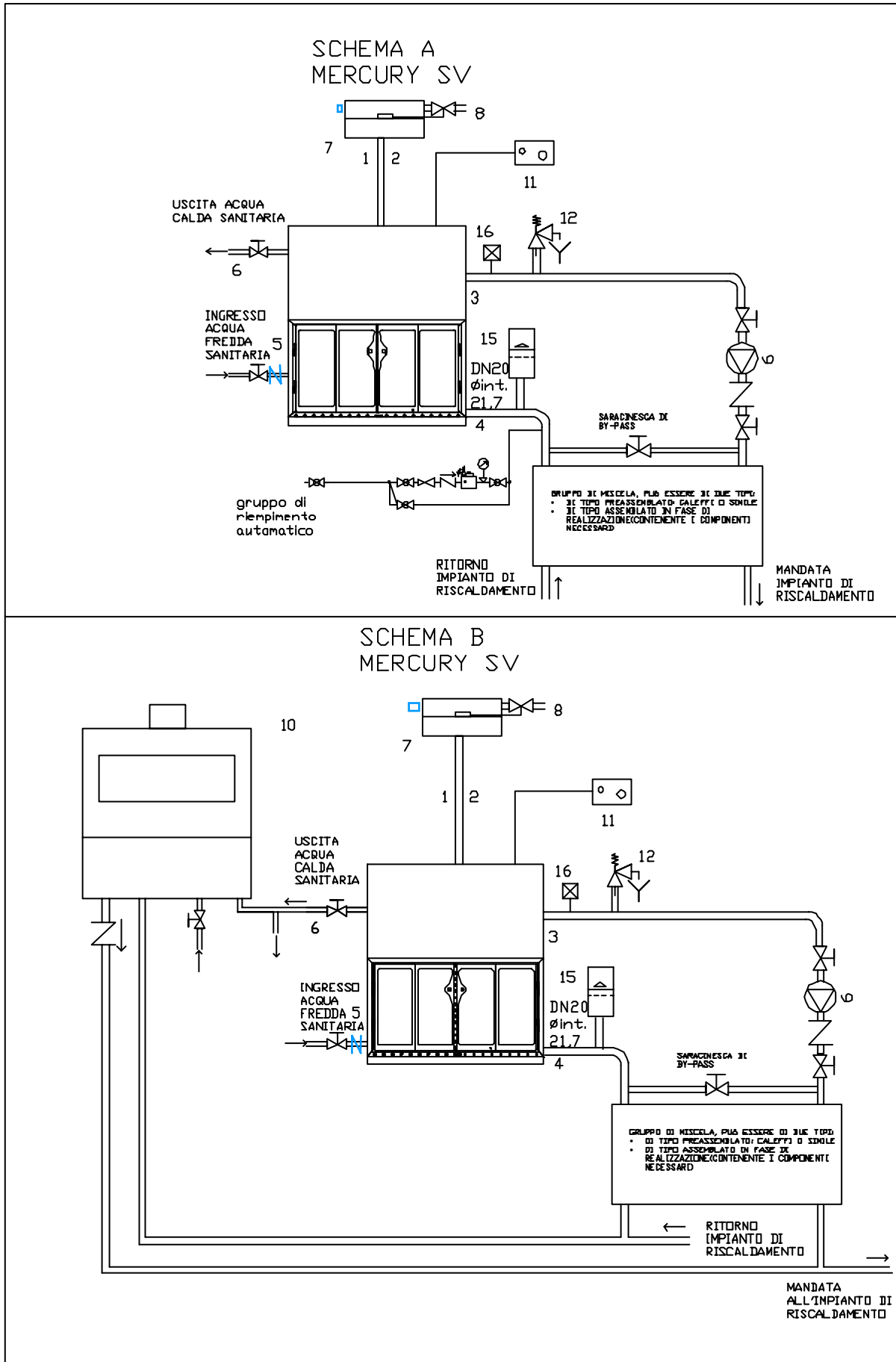
Figura 9 SCHEMA DI COLLEGAMENTO MERCURY 35SV AD IMPIANTO A BASSA TEMPERATURA
