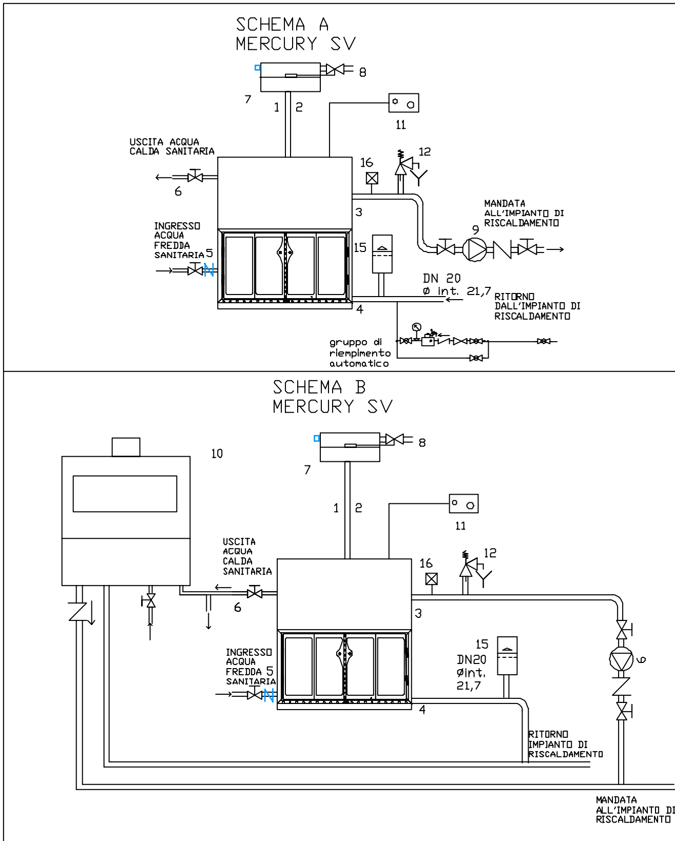
Figura 8 SCHEMA DI COLLEGAMENTO MERCURY 35SV
